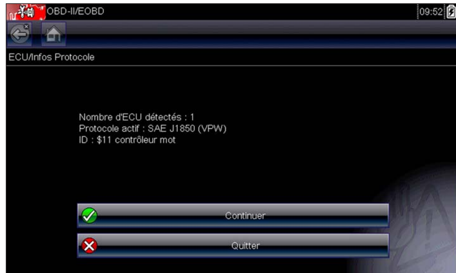
Figure 7-8 Exemple de menu Sélectionner le protocole de communication
