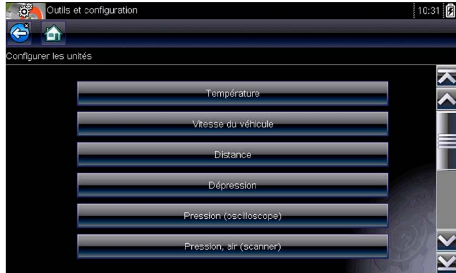
Figure 9-14 Exemple de menu Configurer les unités
